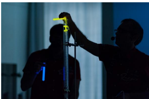
Leuchteffekt: Chemolumineszenz von Oxalsäureestern
